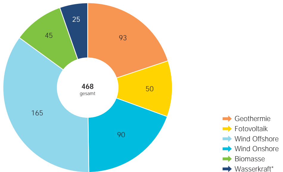
Strommix im Jahr 2050 in Terawattstunden pro Jahr (TWh/a)
