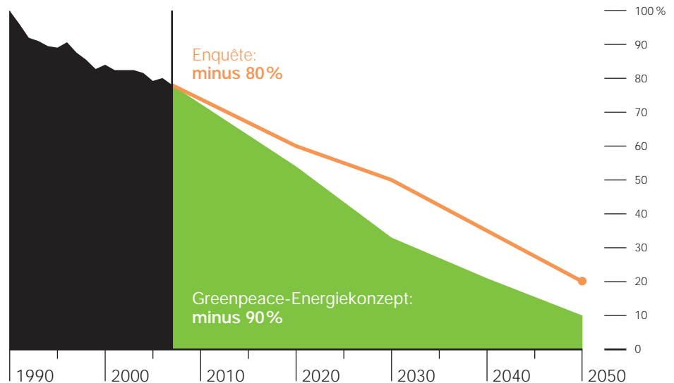
Treibhausgas-Emissionen in Deutschland bis 2050 Empfehlungen der Enquête-Kommission für nachhaltige Energieversorgung (2002) und Greenpeace-Energiekonzept (Basisjahr 1990: 100 Prozent / bis 2007 reale Werte)
